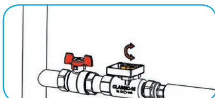
4. Поверните шестерню - сектор для изменения состояния крана
